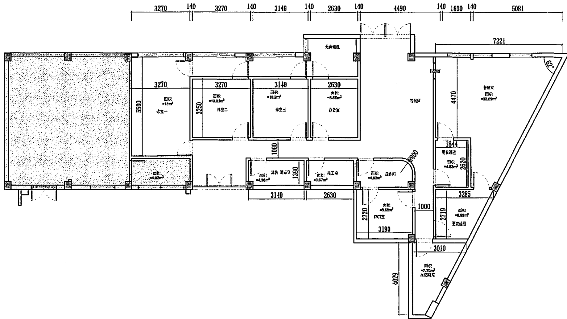
平面布置图
